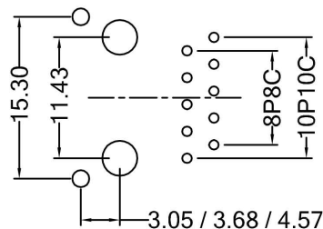
(F3.05) / (F3.68) / (F4.57) PCB LAYOUT / TOP VIEW
